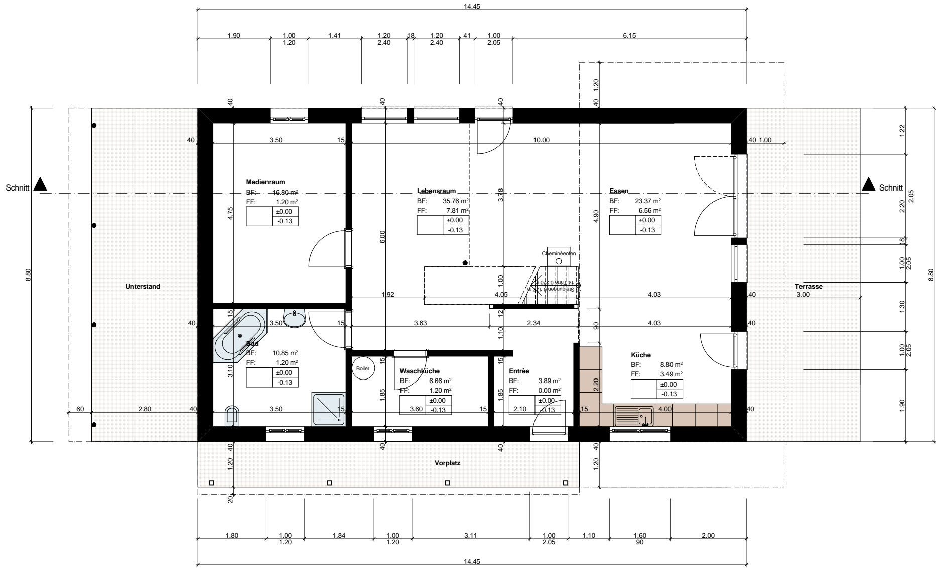
Grundriss Erdgeschoss
